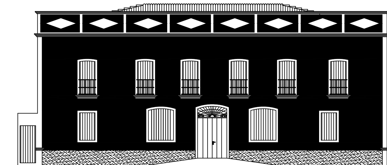
FACHADA FRONTAL
